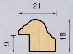
24 / 96 LEGNO/WOOD: AYOUS
