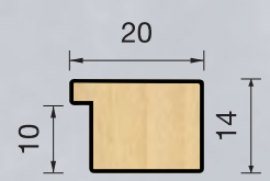
20 / 96 LEGNO/WOOD: AYOUS
